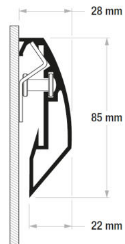
Rahmenquerschnitt
