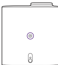
Oberseite Schraubentyp: 1/4" Länge der Schraubenöffnungen: 10mm
