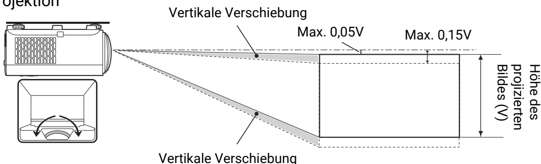
Deckenmontage- Front Projektion
