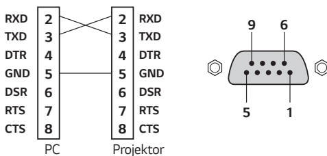
Abbildung 1: RS-232-Verbindungsdiagramm
